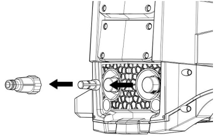
Fig. 12 – Limpieza del filtro de la entrada de agua
