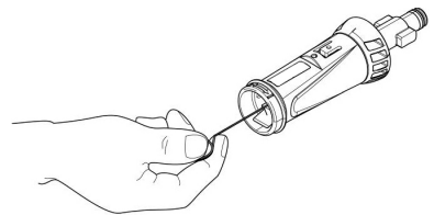
Fig. 13 – Limpeza do bico
