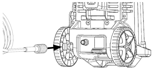
Fig. 6 – Montagem da mangueira no equipamento
