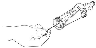
Fig. 12 – Limpeza do bico
