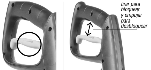
Fig. 10 – Accionamiento del gatillo
